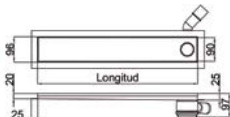
CANAL CON PENDIENTE Y SALIDA EN UN EXTREMO
